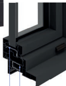
RENFORT 100% Profils acier dans l'ouvrant et le dormant si coloris plaxé 1 ou 2 faces
